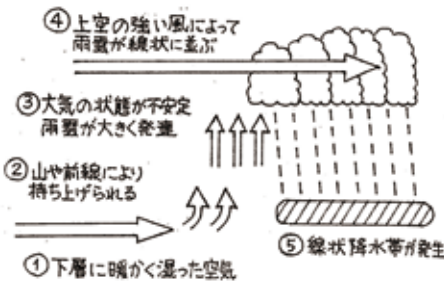
図3 線状降水帯発生メカニズム
